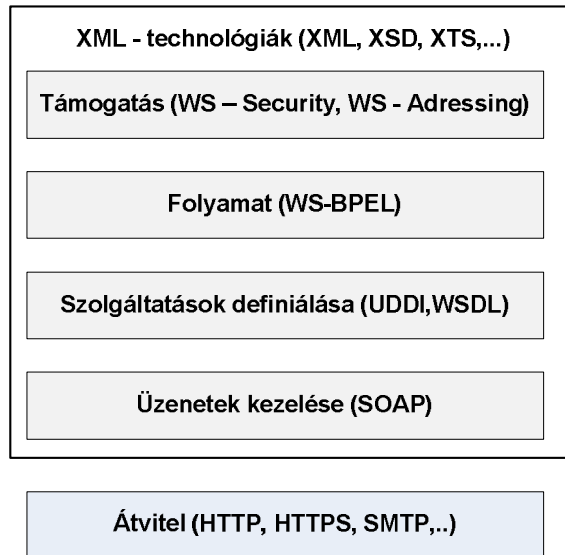
31. ábra. Webszolgáltatás szabványok
