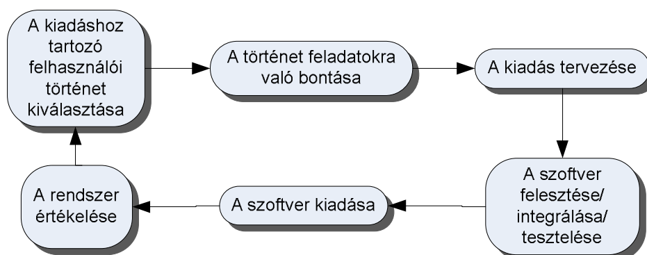
24. ábra: Az extrém programozás kiadási ciklusai
