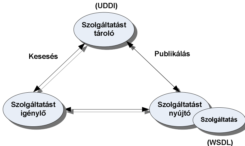
30. ábra. Szolgáltatásorientált architektúra
