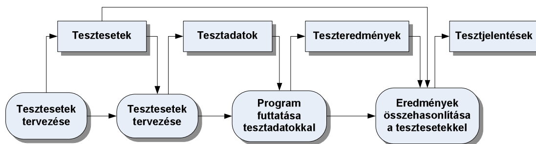
28. ábra. A szoftvertesztelési folyamat modellje
