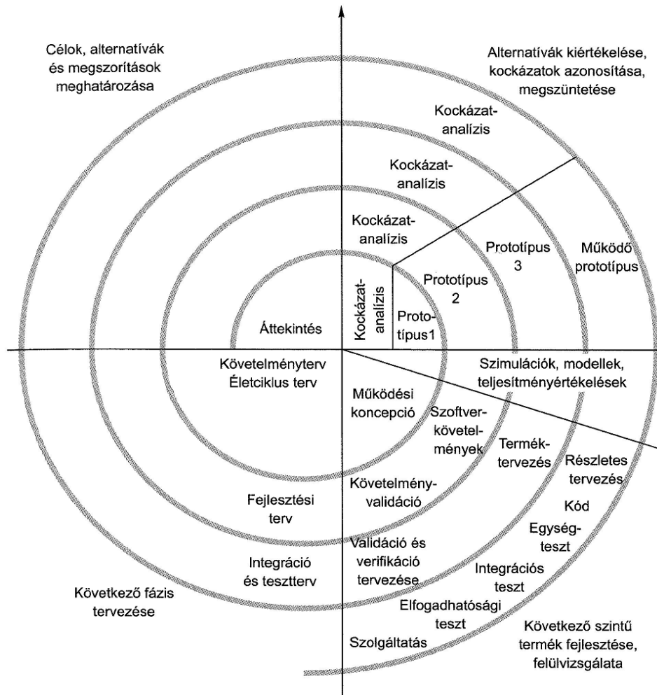
5. ábra. Boehm féle spirálmodell [1]
