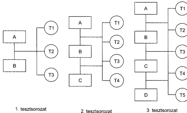
29. ábra. Inkrementális integrációs tesztelés
