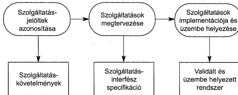
32. ábra. A szolgáltatástervezés folyamata
