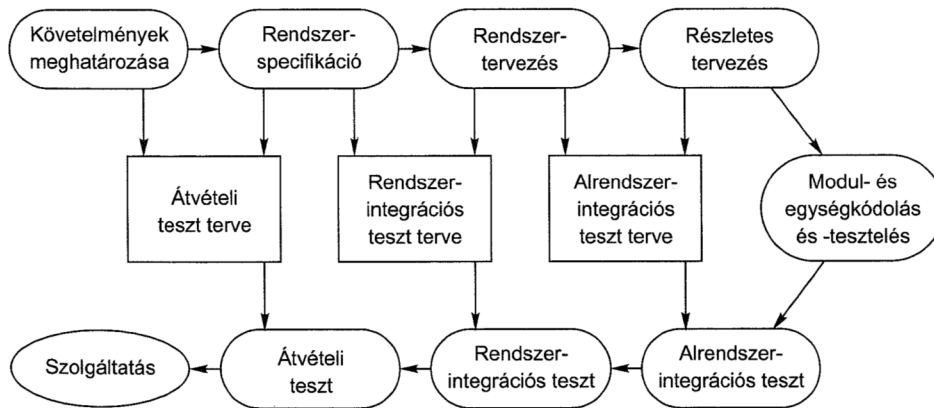
27. ábra. V Modell
