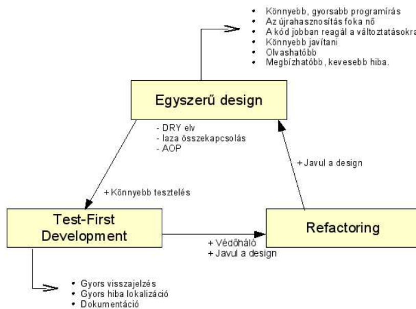
25. ábra: Test Driven Development folyamata
