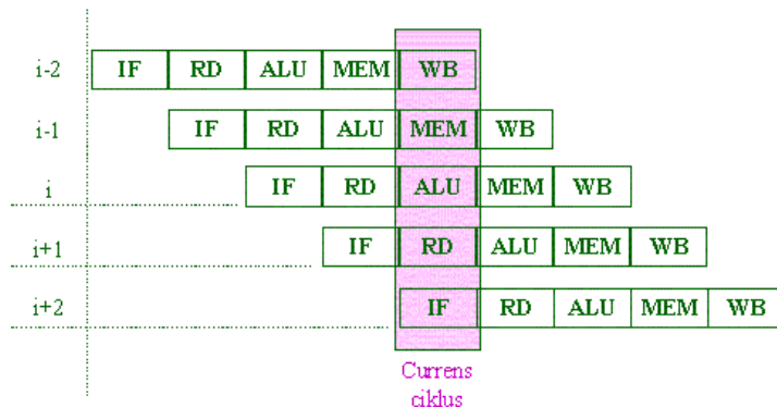
6.2. ábra. Az R3000 5 mélységű csöve
