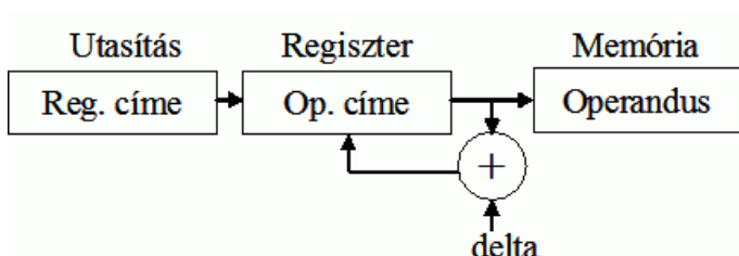
5.7. ábra. Post-auto inkremens címzés
