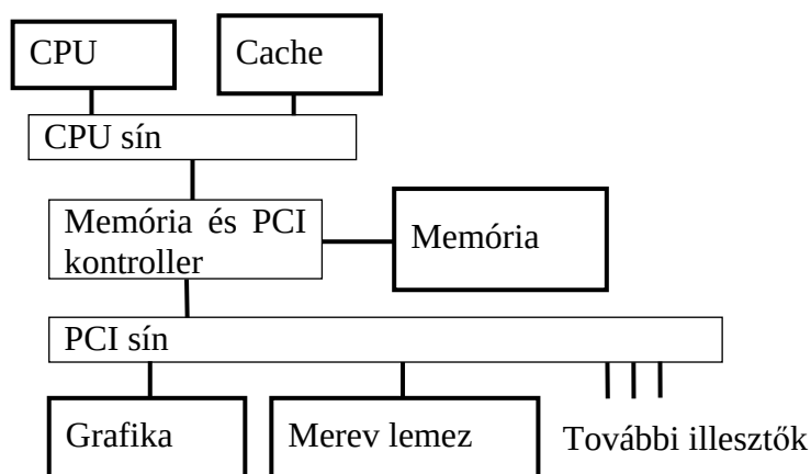
7.3. ábra. PCI sínrendszer
