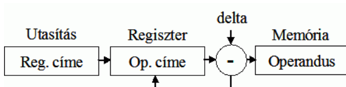
5.5. ábra. Indirekt regiszter címzés
